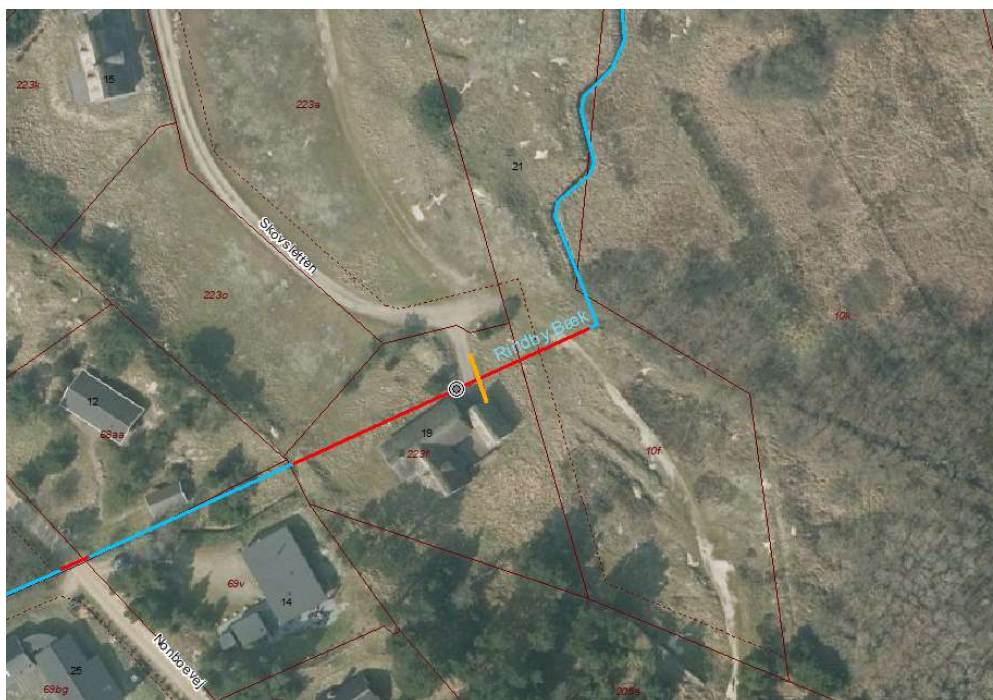
Figur 1: Fiberkablets krydsning af Rindby Bæk i st. 1835 m. Rindby Bæk er vist som en blå og rød streg, hvor den røde streg viser rørlagte strækninger. Den orange linje viser tracéet for den styrede underboring af vandløbet.
